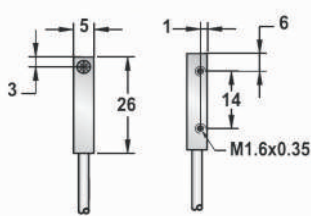
Q5产品尺寸图
