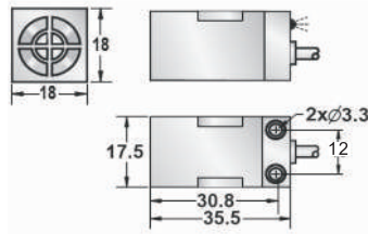
18PQ产品尺寸图
