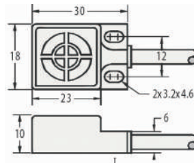
18PQC产品尺寸图
