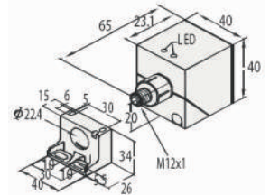
Q40产品尺寸图
